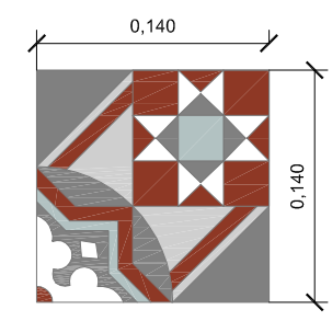
2 LADRILHO GERAL
