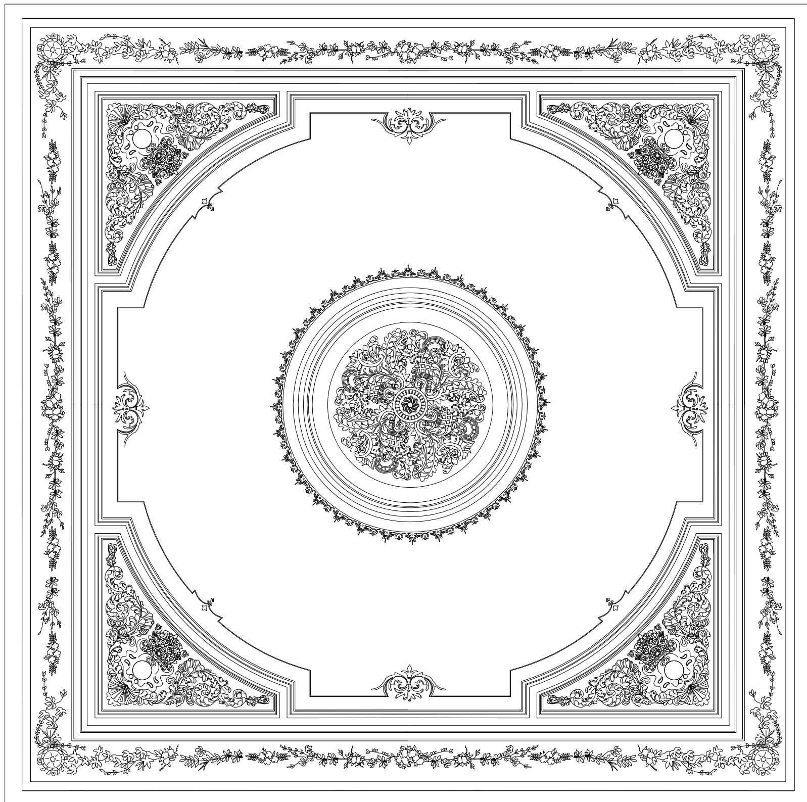
1 PLANTA DE TETO REFLETIDO - SALA PRÓ-ALIADOS
