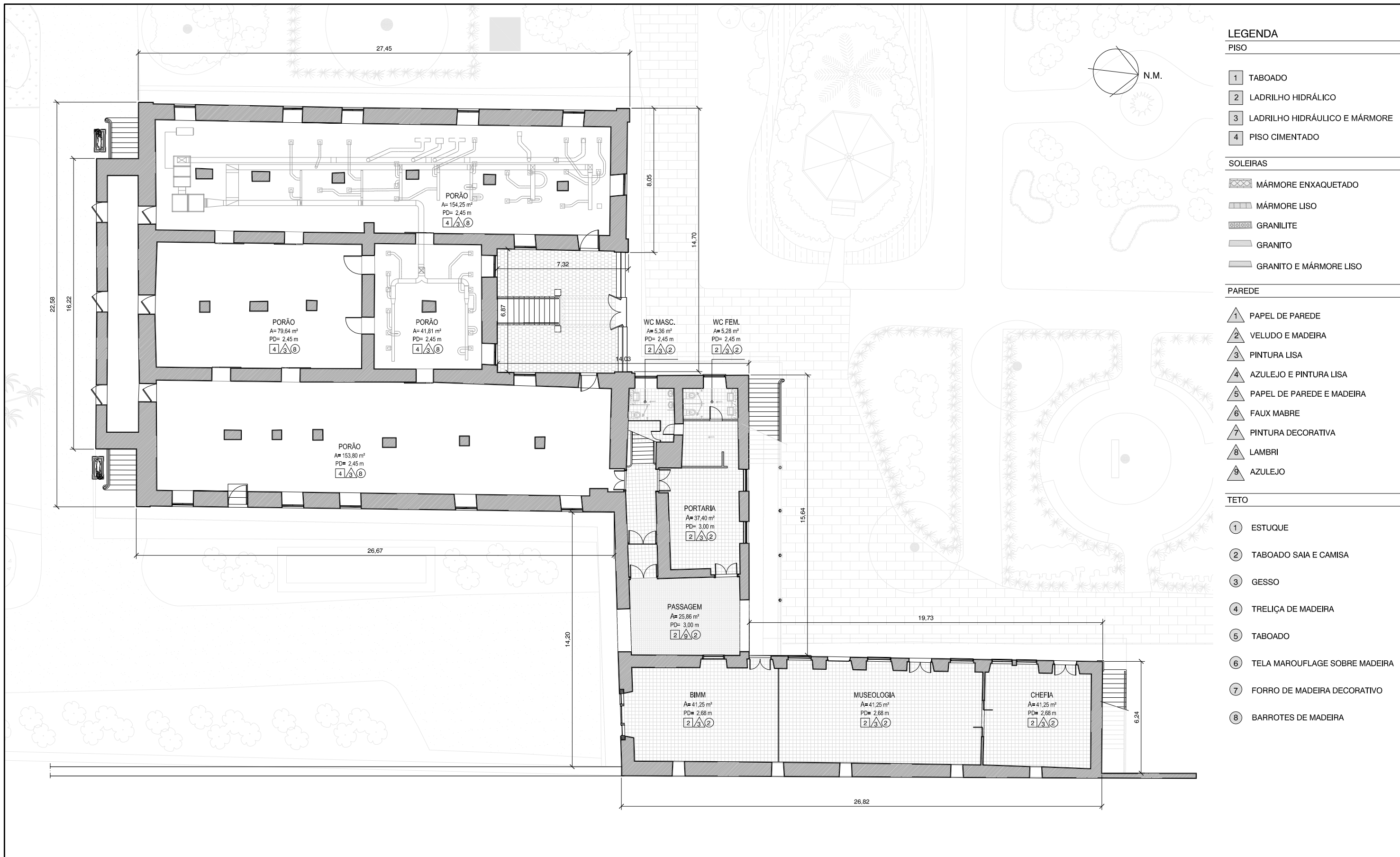
1 PLANTA BAIXA DO PAVIMENTO TÉRREO/PORÃO
