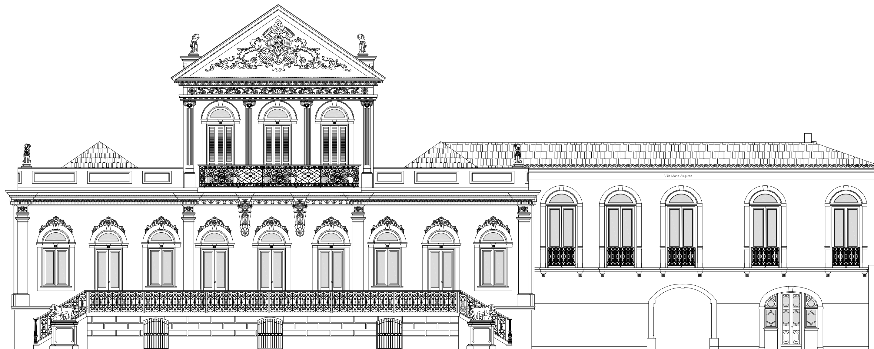
1 FACHADA SUL
