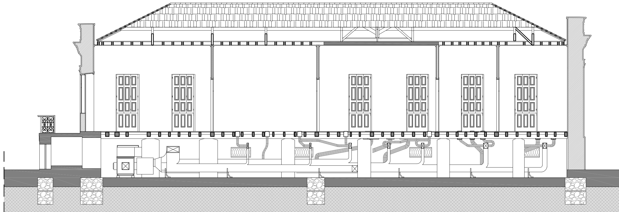
1 CORTE AA
